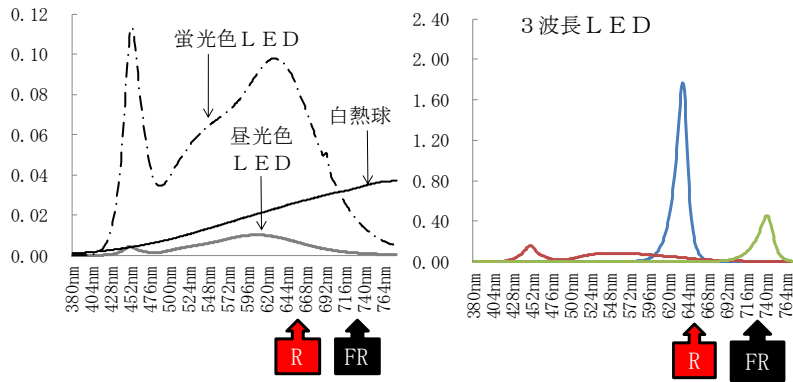
図1 各LED及び白熱球に含まれる波長 注) 単位: 単位エネルギー当たりの相対値。図に示したRは赤色光(660nm)、FRは遠赤色光(730nm)を示した。
